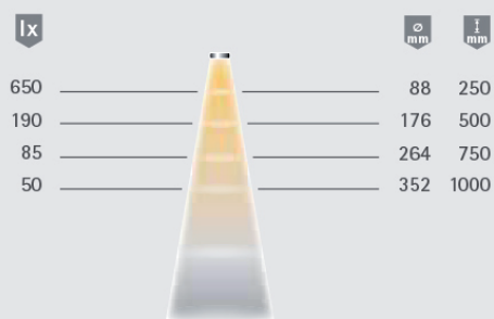
Diagrama de distribución luminosa 20°
